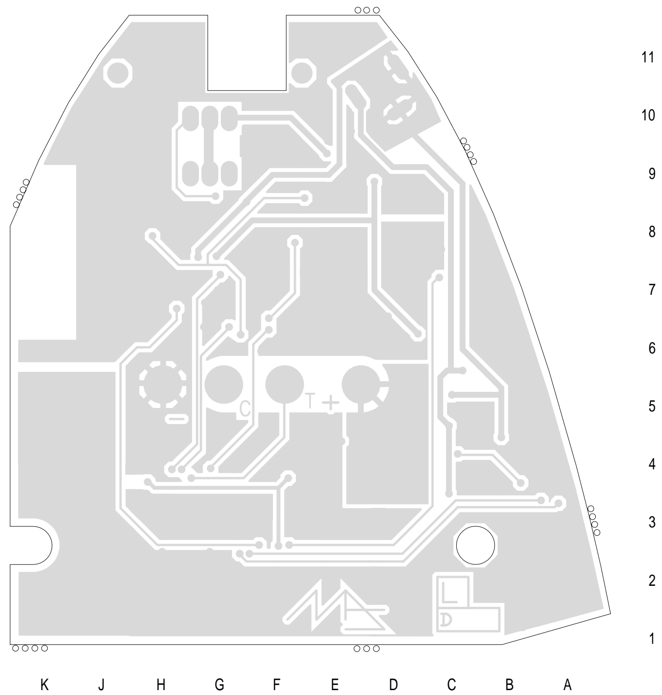
220-01411-00 BOTTOM COPPER
